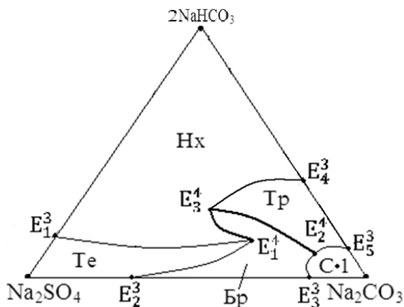
Рис. 2 - Солевая часть диаграммы растворимости системы \text{Na}_2\text{SO}_4\text{-Na}_2\text{CO}_3\text{-NaHCO}_3\text{-H}_2\text{O} при 50^\circ\text{C}
