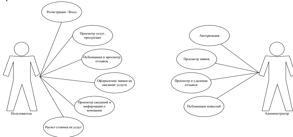
Рис.1 - Диаграмма вариантов использования
