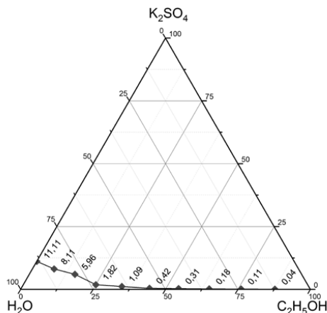
Рис. 3 - Диаграмма растворимости сульфата калия в системе \text{K}_2\text{SO}_4\text{--H}_2\text{O--C}_2\text{H}_5\text{OH} при 25^\circ\text{C}
