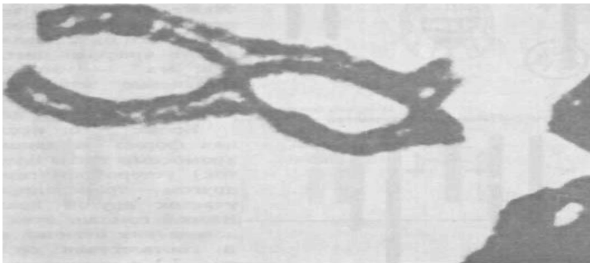
Рис. 1. Хиазмы в диплотене в одном из бивалентов у кузнечика (D. Suzuki, A.Griffiths, R. Levontin, 1981).
