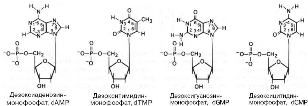
Схема 1. Строение нуклеотидов
