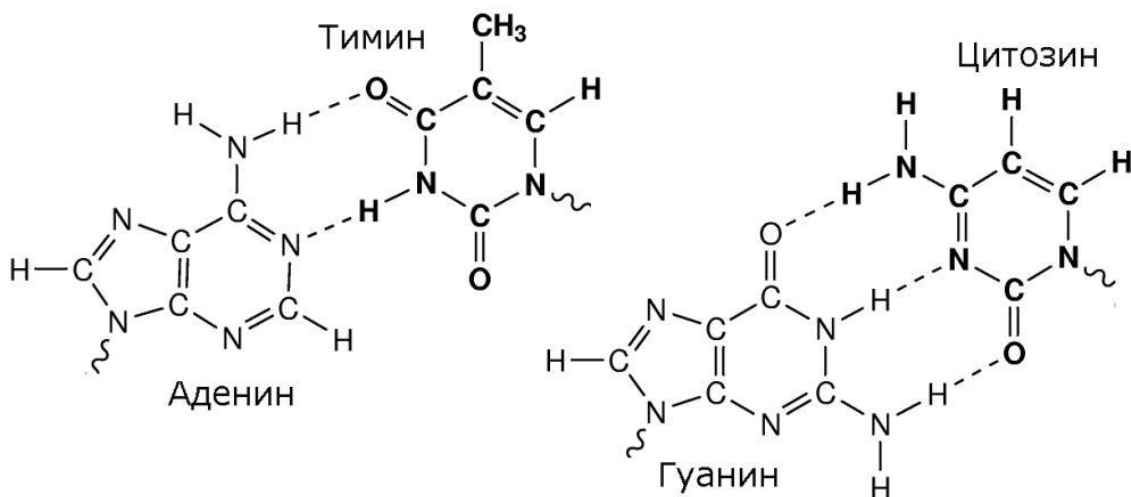
Схема 3. Образование водородной связи между азотистыми основаниями
