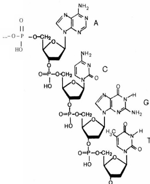
Схема 2. Строение одноцепочечной молекулы ДНК
