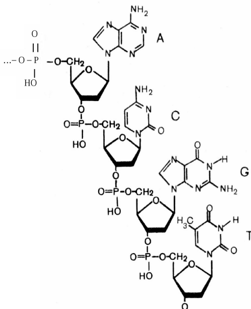
Схема 2. Строение одноцепочечной молекулы ДНК
