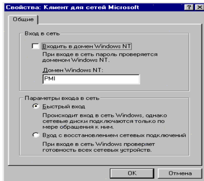
Рисунок 4 – «Свойства»
