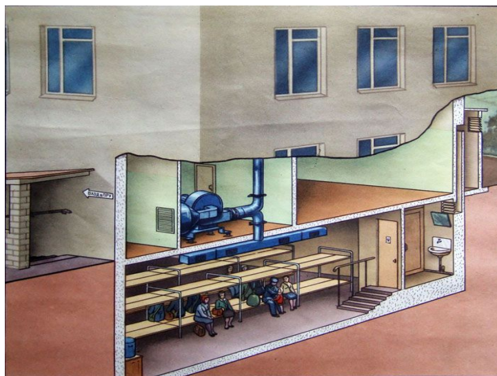
Рис. 6 Встроенное убежище
