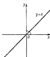
Рисунок 12. График функции y=kx
