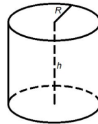
Рисунок 82. Цилиндр
