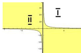
Рисунок 28. График функции y=4/x
