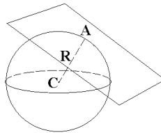
Рисунок 74. Касательная плоскость к сфере
