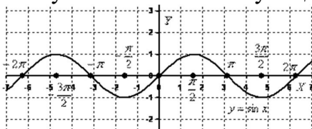
Рисунок 19. График функции y=\sin x
