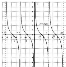
Рисунок 22. График функции y = \operatorname{ctg} x
