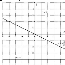
Рисунок 3. Частные случаи графика линейной функции
