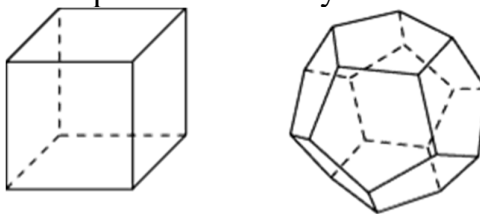
Рисунок 70. Правильные многогранники
