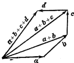
Рисунок 38. Правило многоугольника
