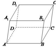
Рисунок 53. Параллелепипед
