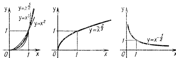
Рисунок 15. Графики степенных функций
