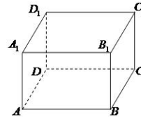
Рисунок 54. Прямоугольный параллелепипед
