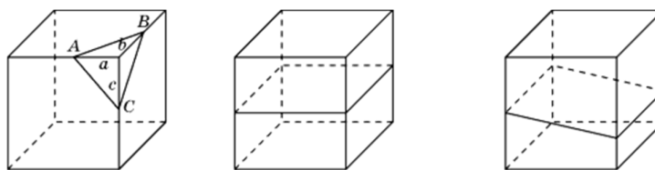
Рисунок 55. Сечения куба плоскостью
