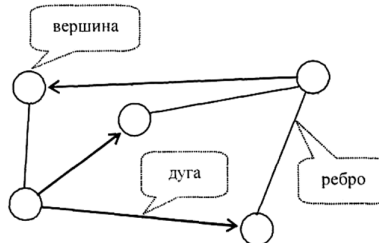
Рис. 1. Пример графа
