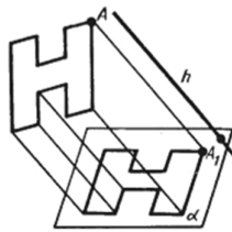
Рисунок 51. Изображение пространственных фигур на плоскости
