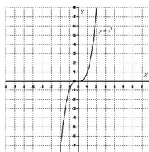
Рисунок 6. График функции y=x^3
