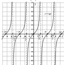
Рисунок 21. График функции y = \operatorname{tg} x
