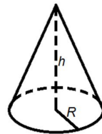
Рисунок 83. Конус
