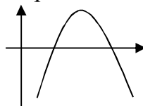
Рисунок 10. Эскиз графика
