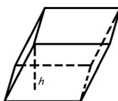
Рисунок 78. Параллелепипед
