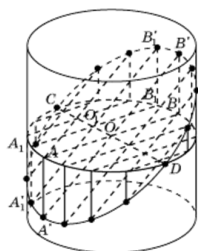
Рисунок 63. Сечение цилиндра
