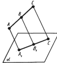
Рисунок 52. Изображение отрезка на плоскости
