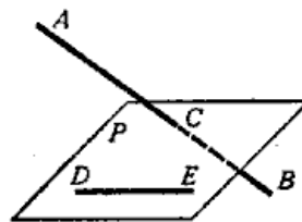
Рисунок 40. Непересекающиеся прямые
