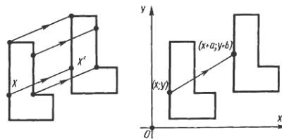
Рисунок 45. Параллельный перенос
