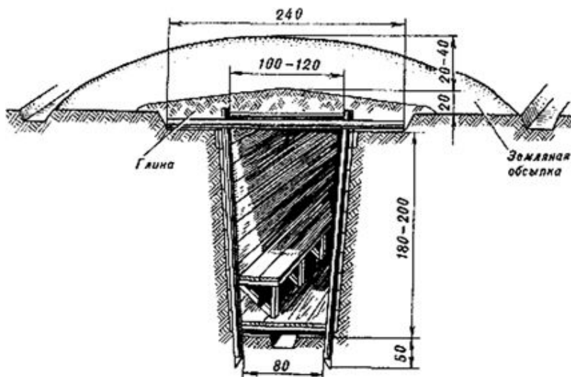
Рис. 9. Устройство «Щели»
