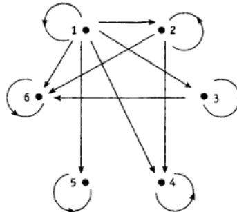
Рисунок 1. Отношение R на множестве A .
