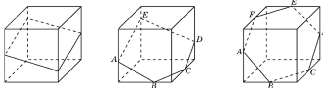
Рисунок 56. Сечения куба плоскостью
