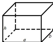
Рисунок 79. Прямоугольный параллелепипед
