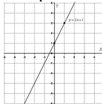
Рисунок 2. График функции y=2x+1
