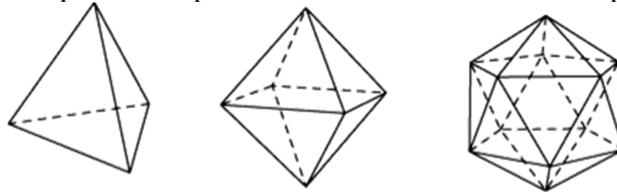
Рисунок 69. Правильные многогранники
