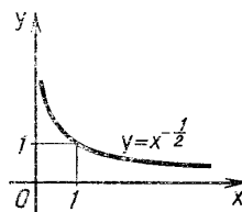
Рисунок 16. График функции y = x^{-\frac{1}{2}}
