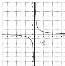
Рисунок 8. График функции y = \frac{1}{x}
