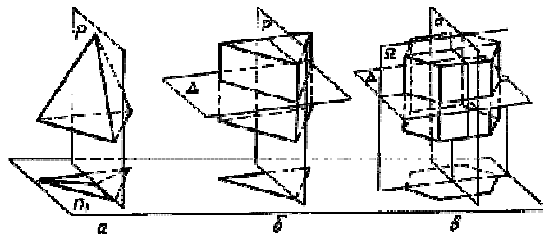
Рисунок 47. Плоскости симметрии
