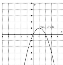
Рисунок 5. График функции y=-x^2+2x
