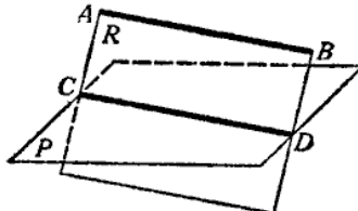
Рисунок 41. Прямая и плоскость параллельные между собой
