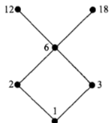
Рисунок 2. Диаграмма Хассе.
