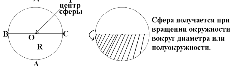
Рисунок 72. Сфера
