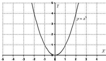
Рисунок 4. График функции y=x^2
