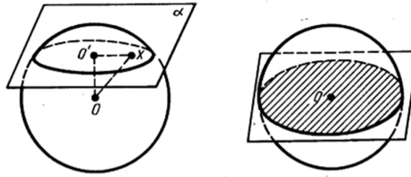
Рисунок 75. Сечение шара
