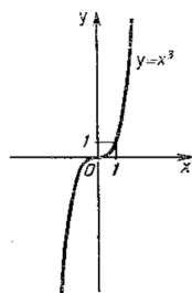
Рисунок 14. График функции y=x^3
