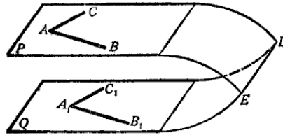
Рисунок 44. Параллельные плоскости
