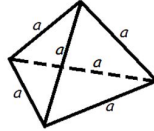
Рисунок 81. Тетраэдр
