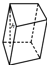
Рисунок 77. Призма
