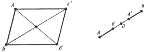
Рисунок 46. Параллельный перенос
