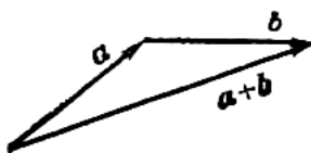
Рисунок 36. Правило треугольника
