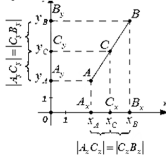
Рисунок 33. Координаты середины отрезка
