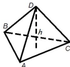
Рисунок 80. Пирамида
