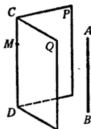
Рисунок 42. Параллельность прямой линии пересечения плоскостей
