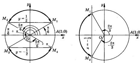
Рисунок 1. Решение тригонометрического неравенства.
