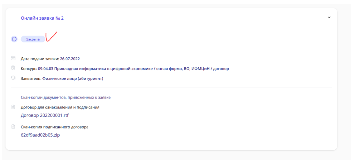
Рисунок 24. Заявка закрыта
