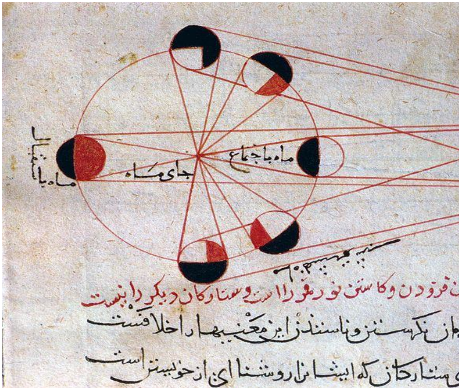
ФАЗЫ ЛУНЫ. ЧЕРТЕЖ АЛЬ-БИРУНИ, 11 ВЕК.
