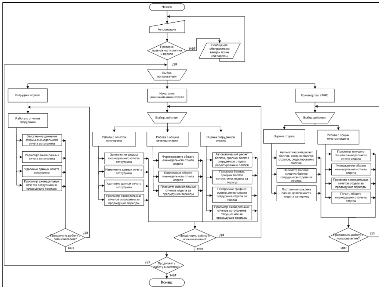
Рис. 5. Пример блок-схемы алгоритма работы программы
