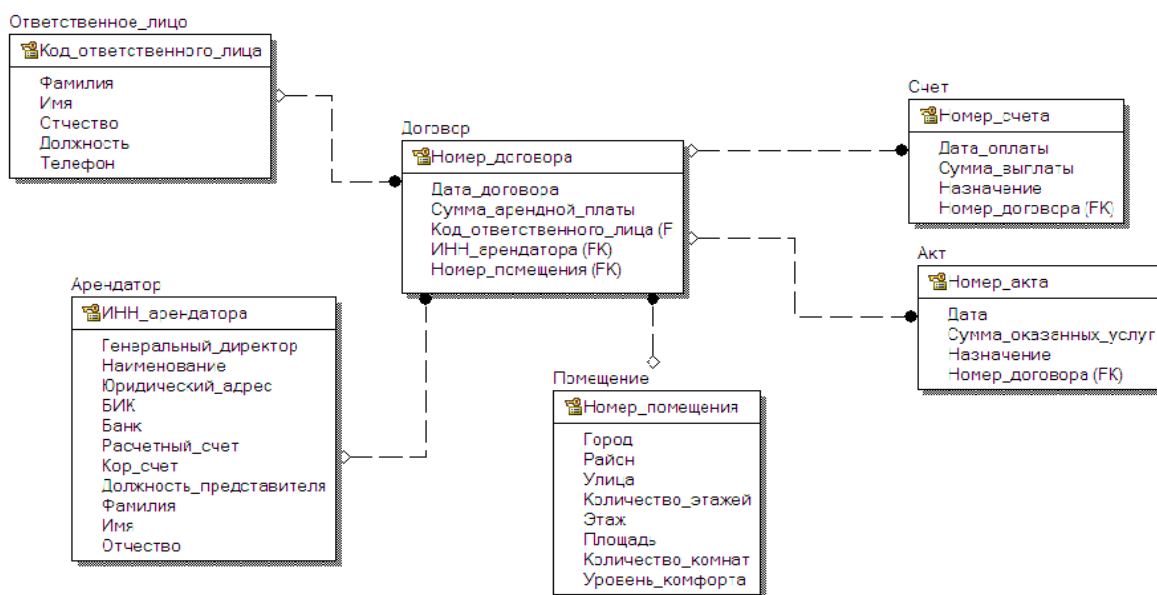
Рис 1. Пример информационной модели
