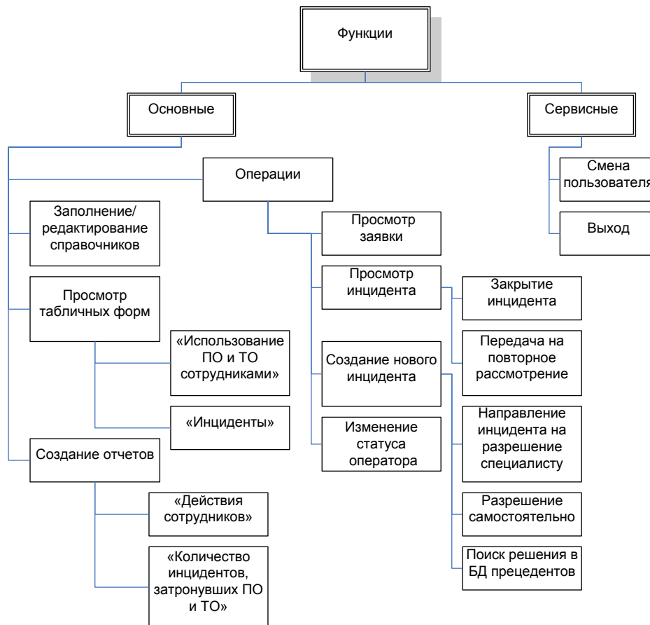
Рис. 2. Пример дерева функций
