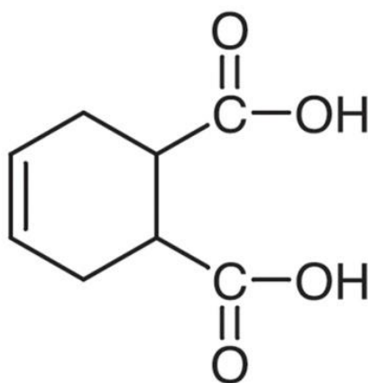
цис -циклогексен-1,2-дикарбоновая кислота
