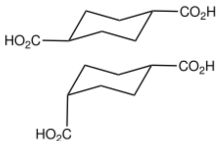
1,4-циклогександикарбоновая кислота
