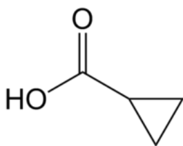
циклопропанкарбоновая кислота
