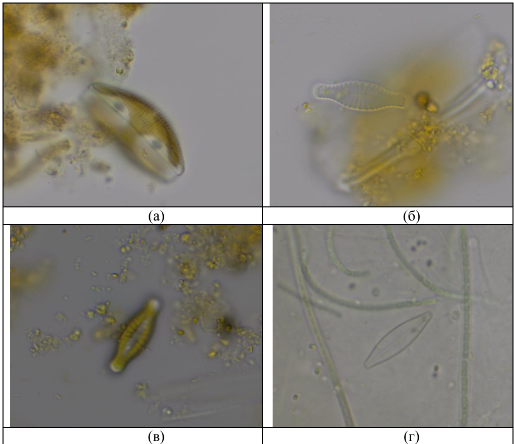
Рис. 3. Водоросли пруда в Салихово: (а) Cymbella sp, (б) Fragilaria construens , вид с середины клетки, в) Navicula lanceolate , вид сверху, (г) Navicula lanceolata
