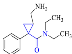
(a) Levomilnapiaran (Antidepressant)
