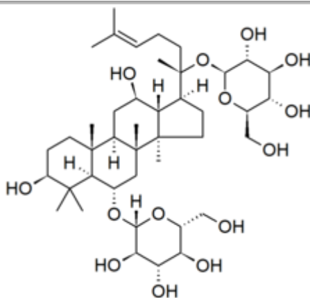
гинсенозид Rg1
