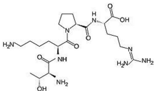
тафтсин
