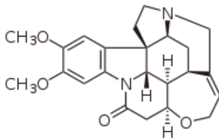
бруцин
