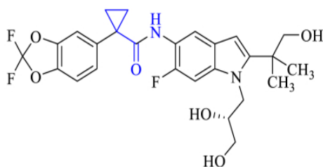
(d) Tezacaftor (To treat Cystic fibrosis)
