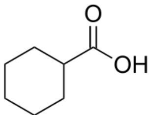
циклогексанкарбоновая кислота
