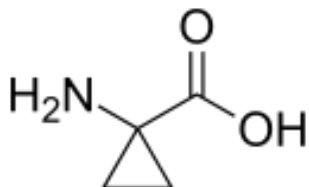
1-аминоциклопропановая кислота
